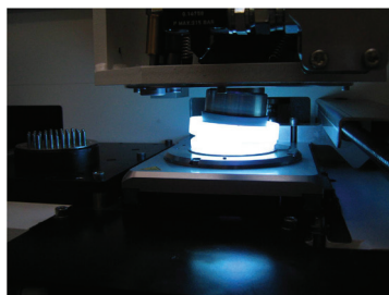
Satisloh公司利用Phoseon公司的UV LED光固化灯研发了On-Block技术
